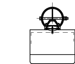
ボックス取付部拡大図 (1/10)
